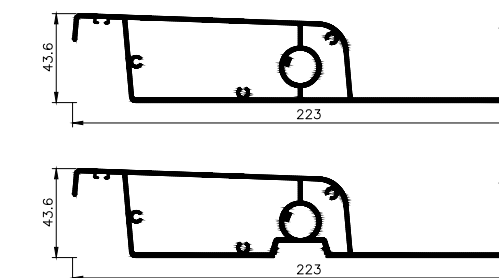
44×223 mm roof slats
